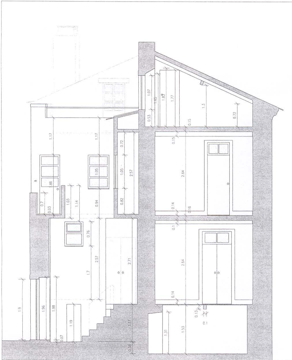
CORTE DD
