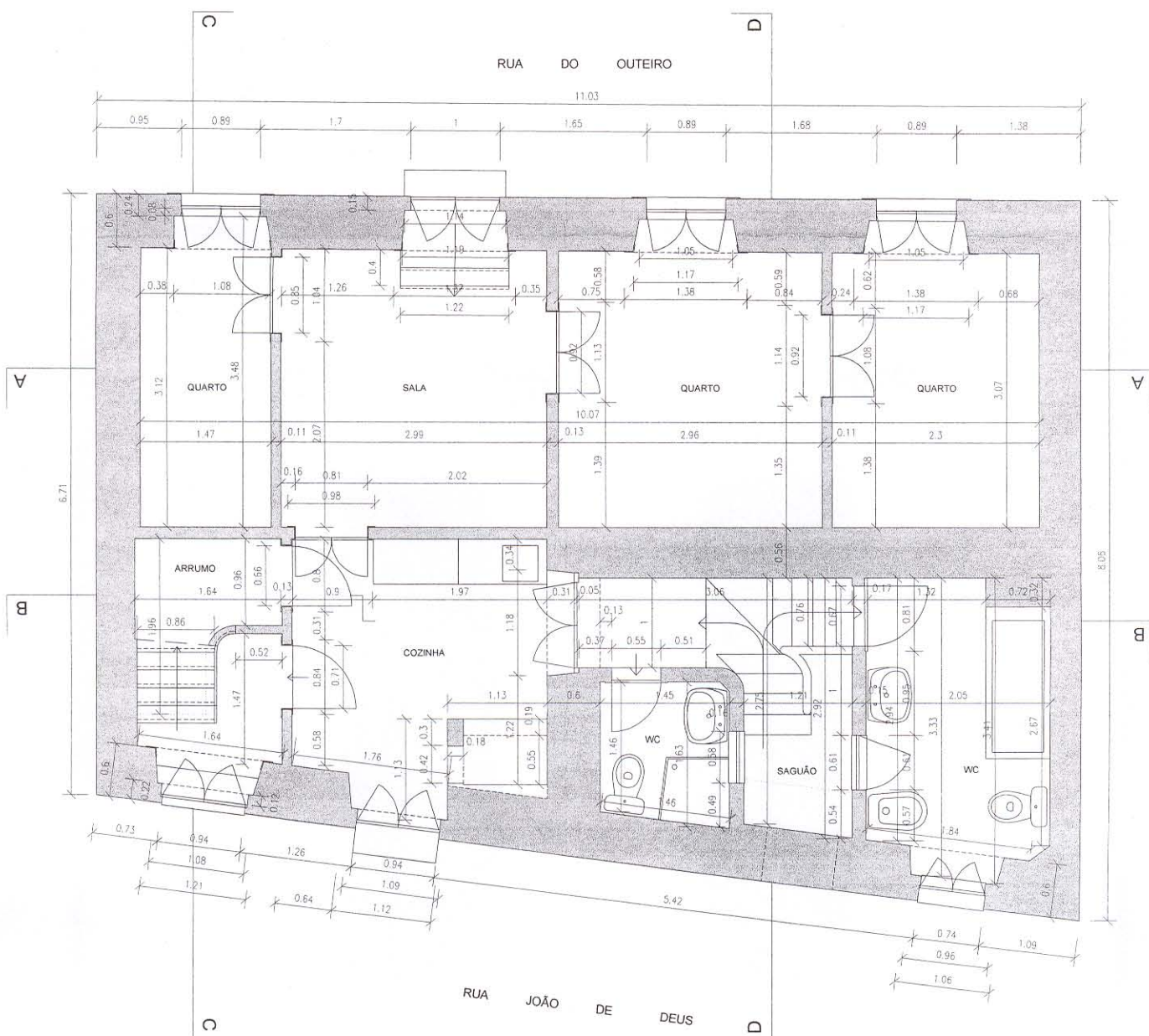
PISO 0 - PLANTA DO R/C
