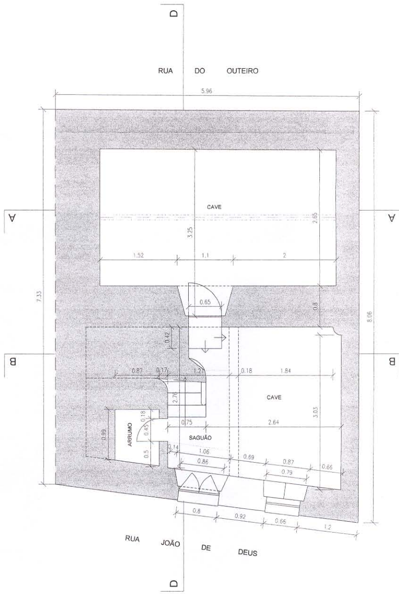
PISO -1 - PLANTA DA CAVE
